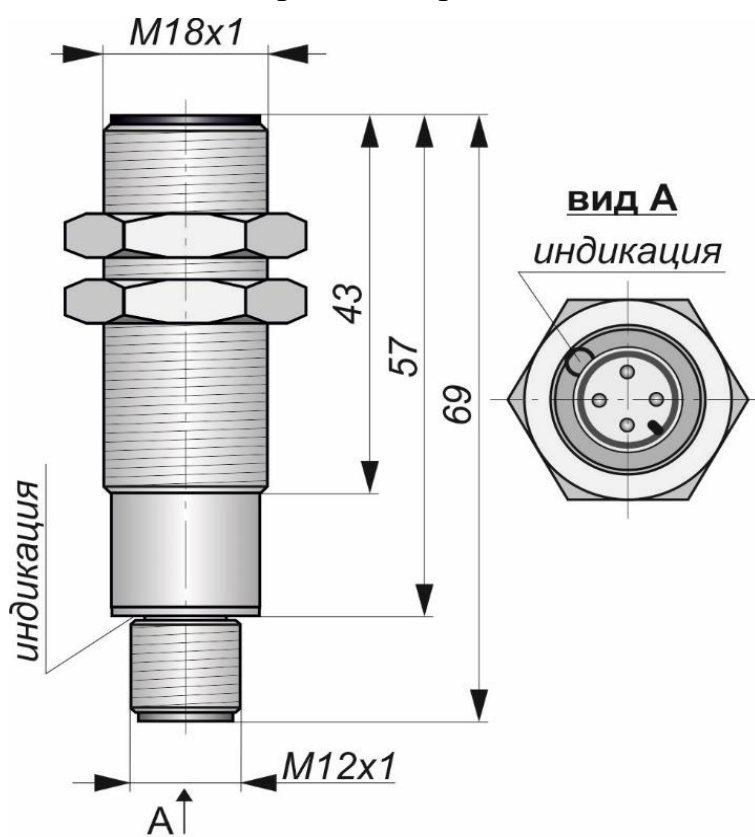
Габаритный чертеж
